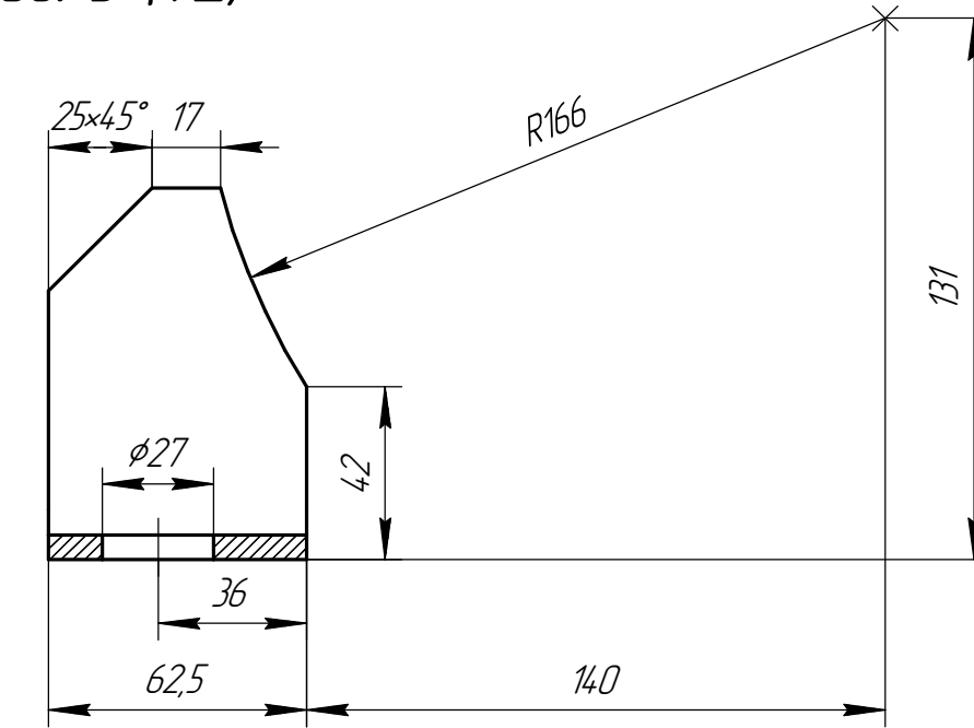
Дет. поз. 3 (1:2)
