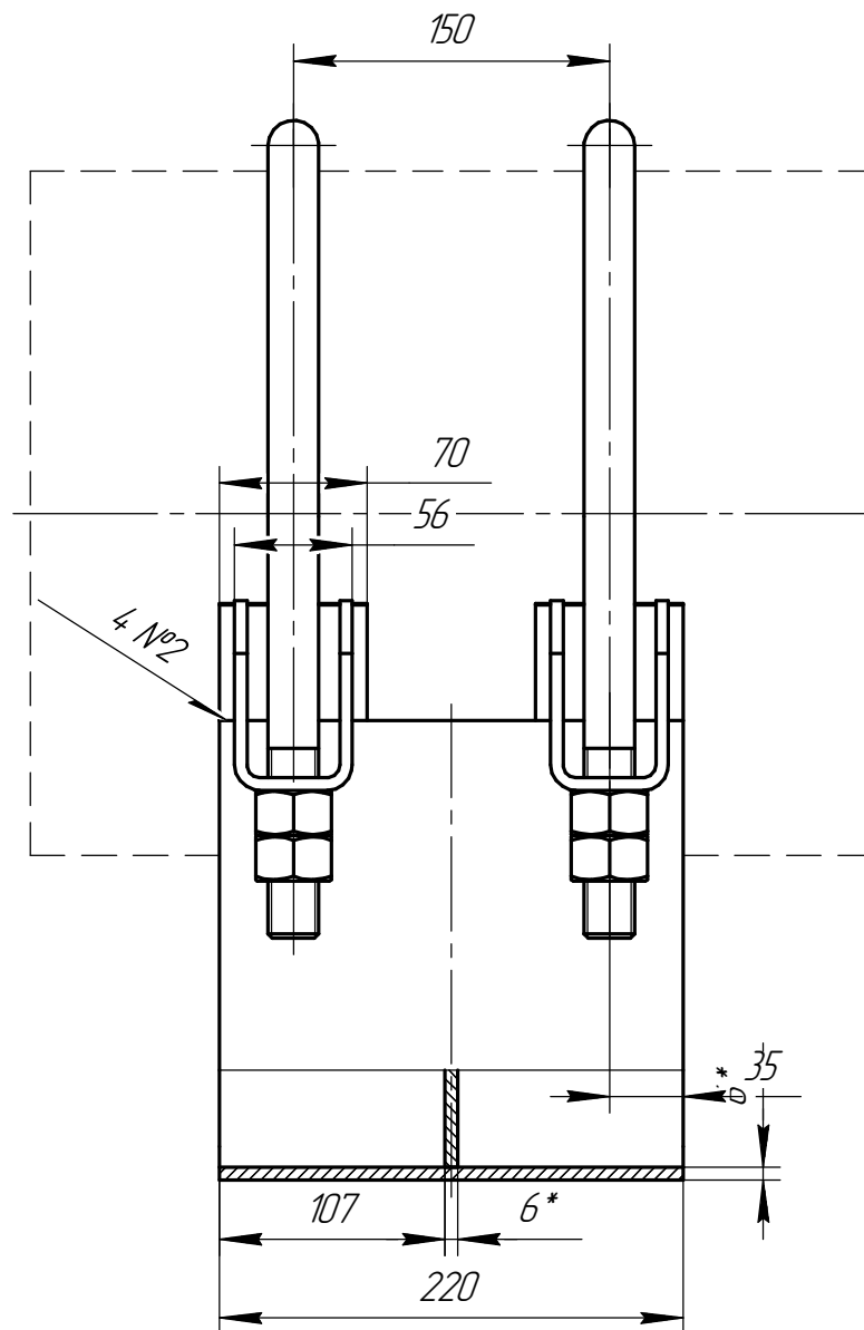
Дет. поз. 4
