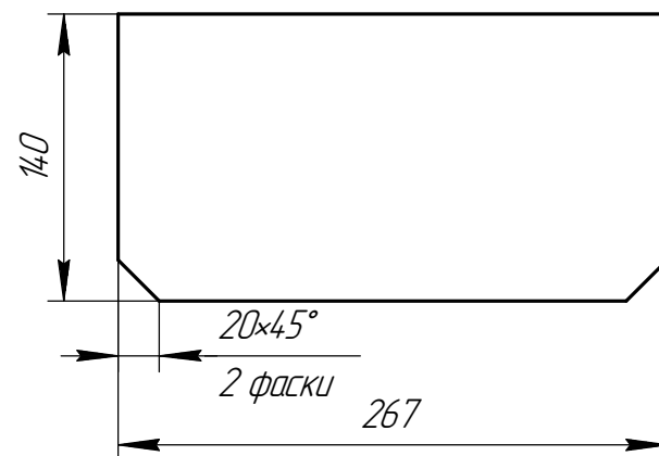
Дет. поз. 2
